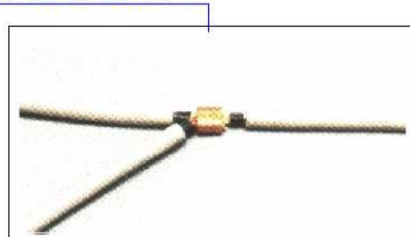
CRIMPATURA DEI CONDUTTORI
