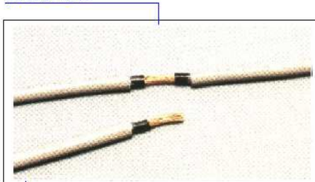
LINEA IN DERIVAZIONE FG7R 1x2.5mmq
