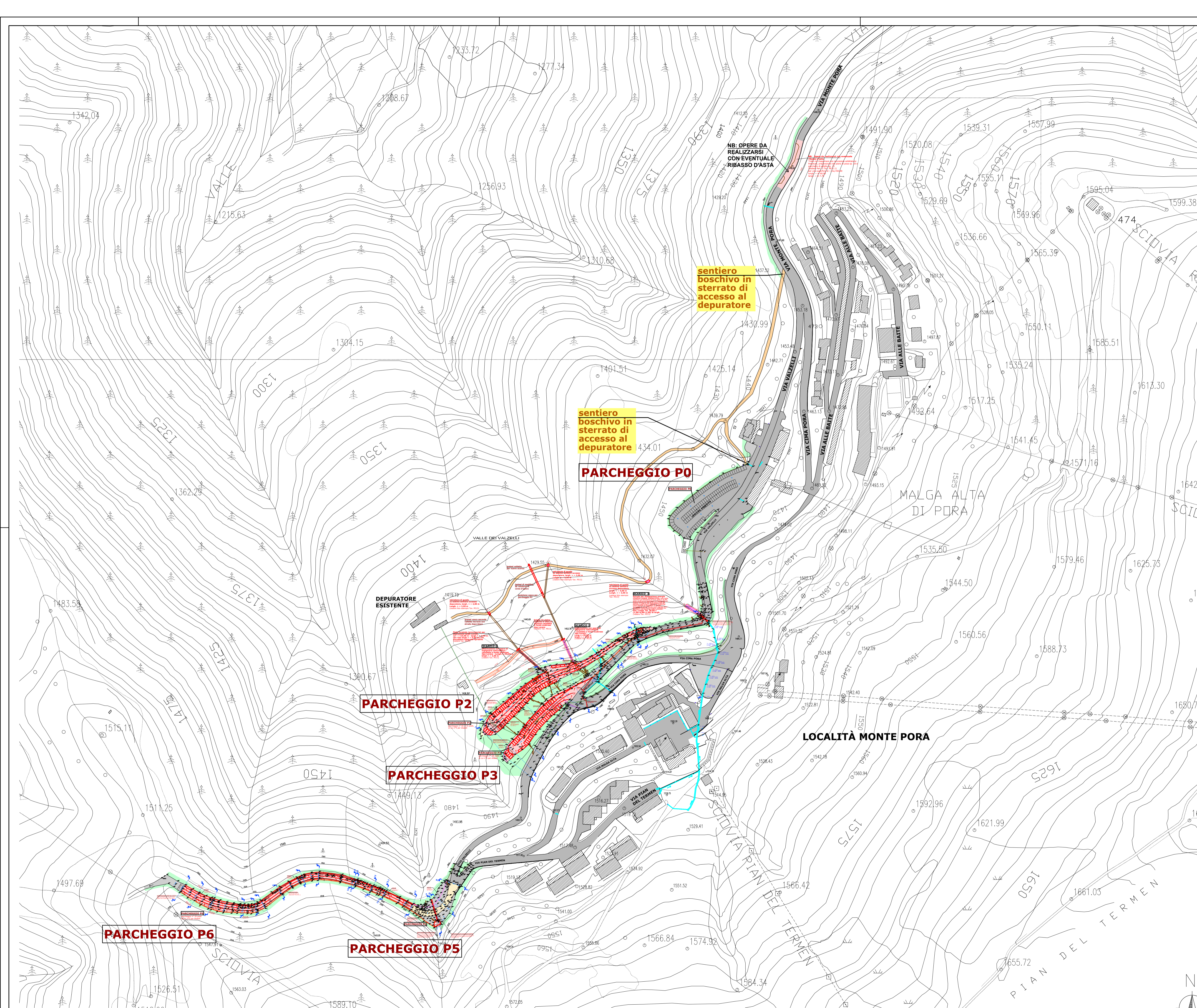
PLANIMETRIA GENERALE - STATO DI PROGETTO CON SOVRAPPOSIZIONE (1:2.000)
